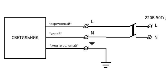
Рисунок 1. Электрическая схема подключения.
